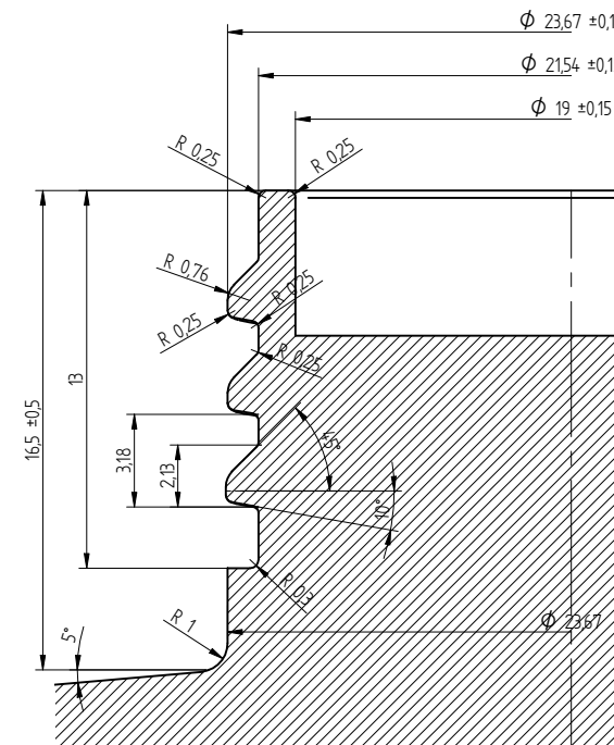
Przekrój A-A 51
