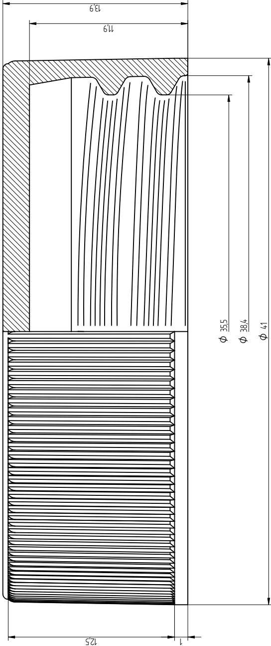
PRZĘKRÓJ B-B 5:1
