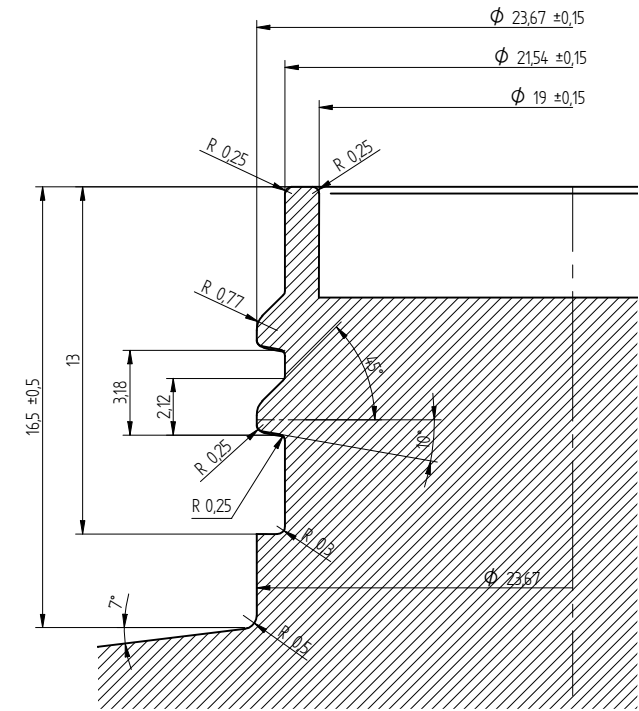
Przekrój A-A 51
