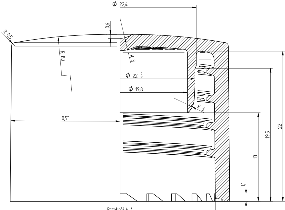
Przekrój A-A 5.1
