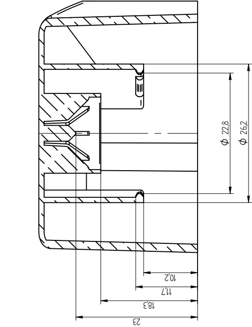
Przekrój C-C
