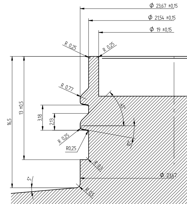
Przekrój A-A 51
